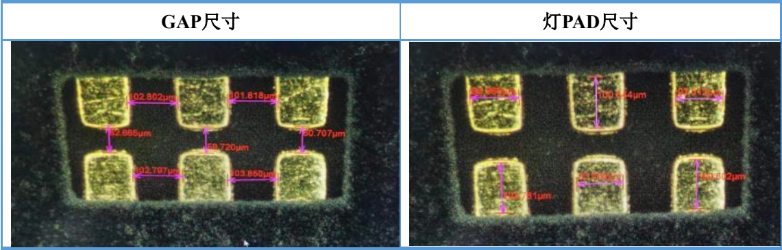
GAP 与灯 PAD 尺寸数据
