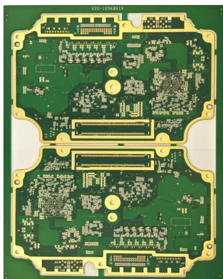
八层化金板
