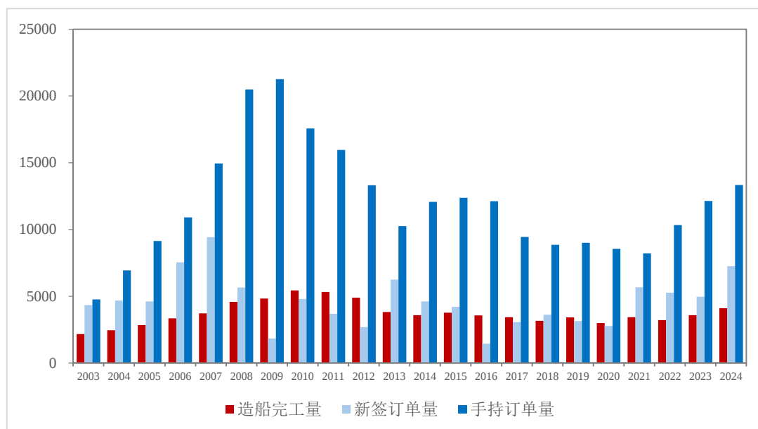
全球造船三大指标
