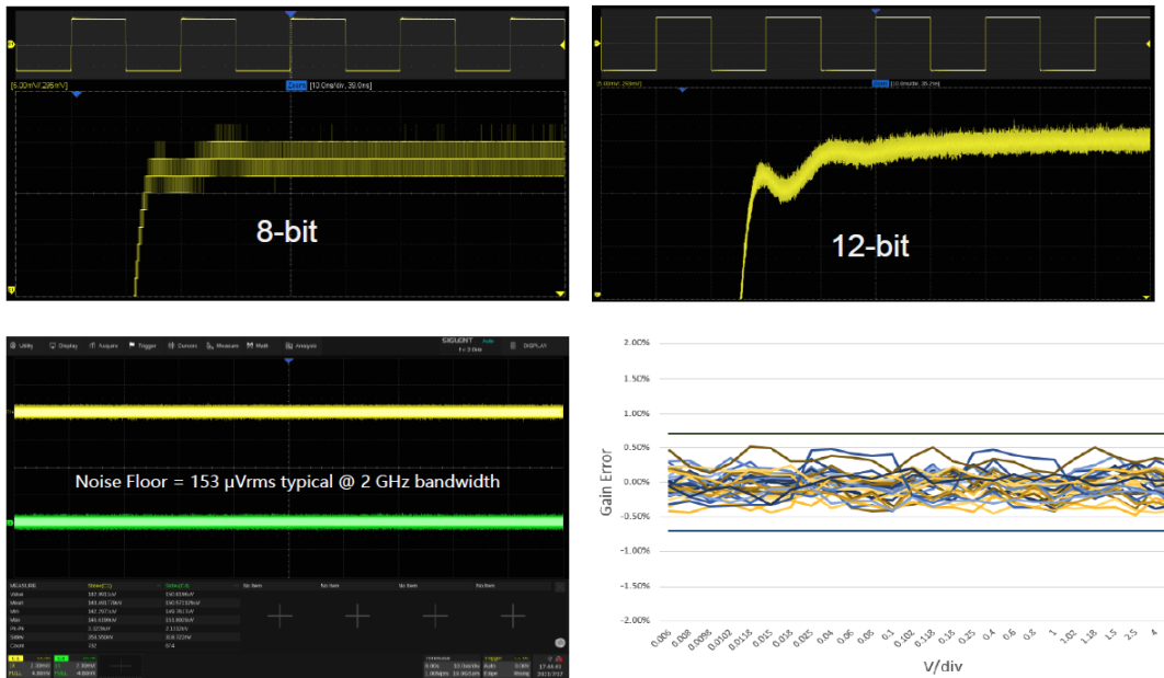
图 1 SDS6000 Pro 12-bit 同 8-bit 对比以及领先所有国内同行的 153 \mu Vrms 底噪
