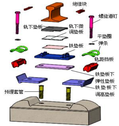
扣件系统组装图——以 WJ-8 型高铁扣件为例
