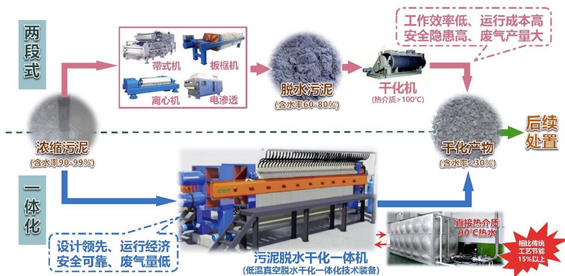
污泥脱水干化“两段式”与低温真空“一体化”工艺对比示意图
