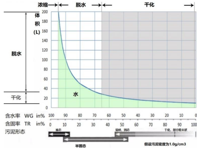
污泥重量、体积与含水率的关系
