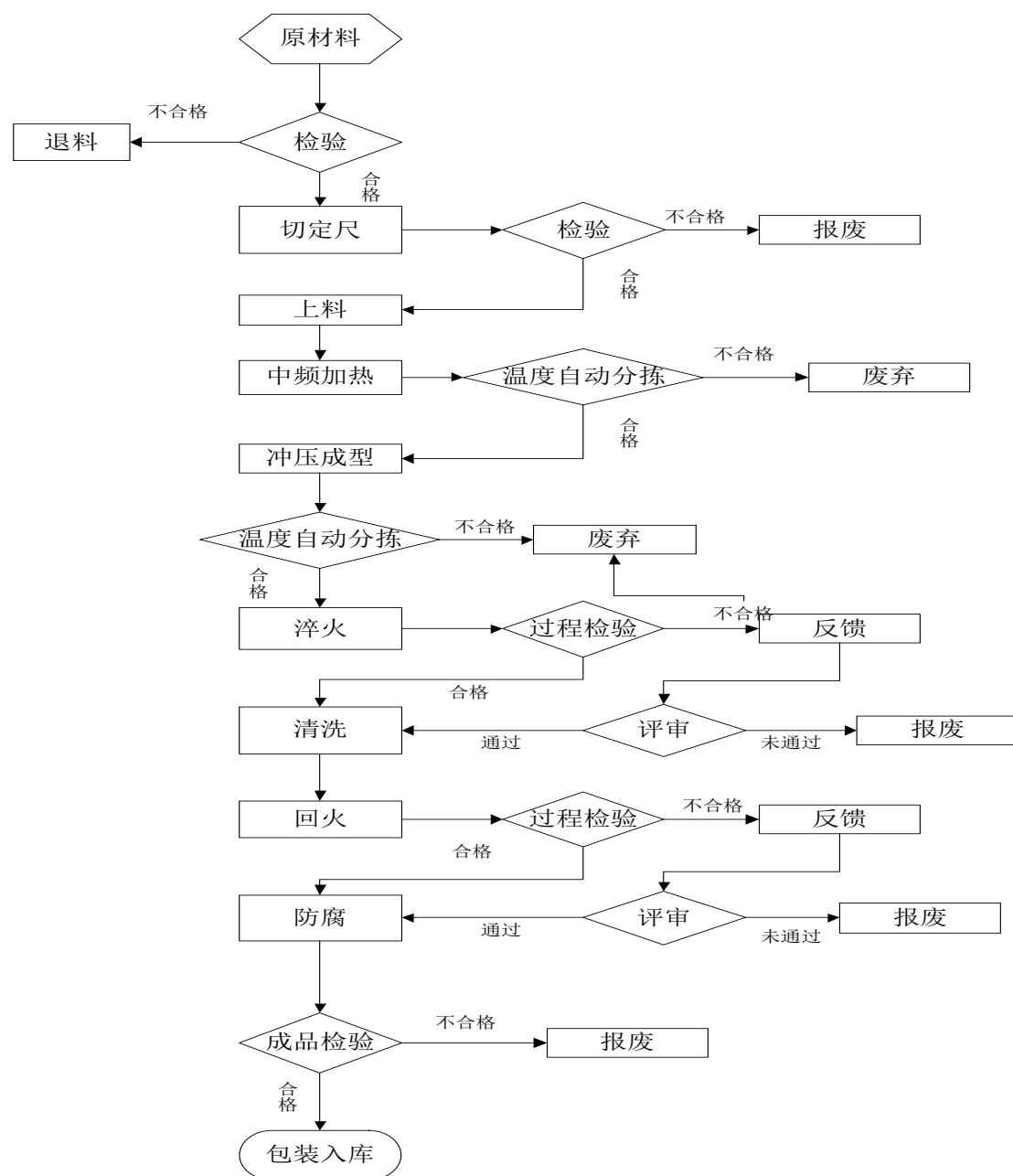
(1) 弹条工艺流程图
