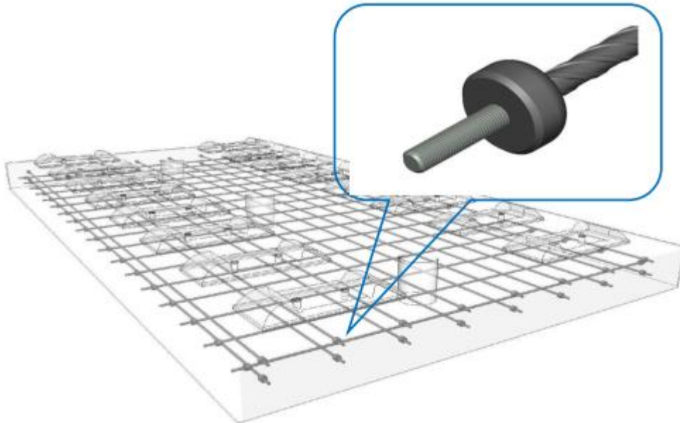
CRTSIII无砟轨道板预应力体系示意图
