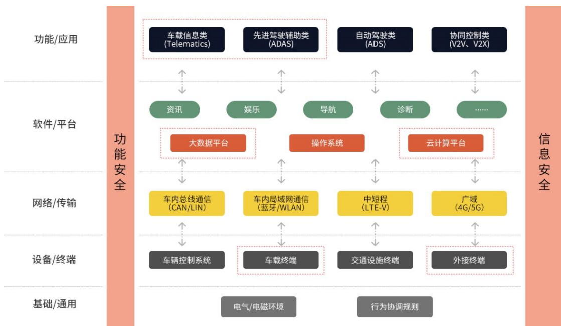
图、智能网联汽车产品物理结构
