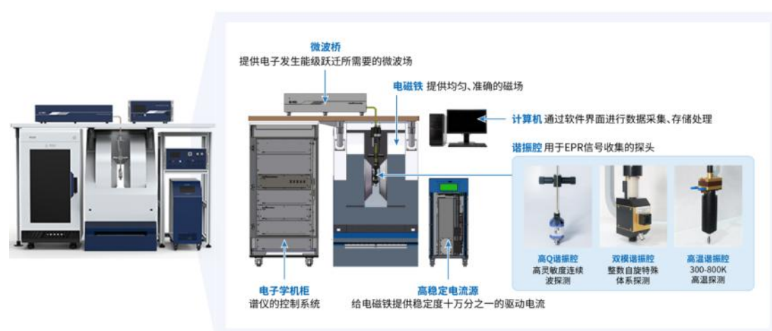
电子顺磁共振波谱仪结构示意图
