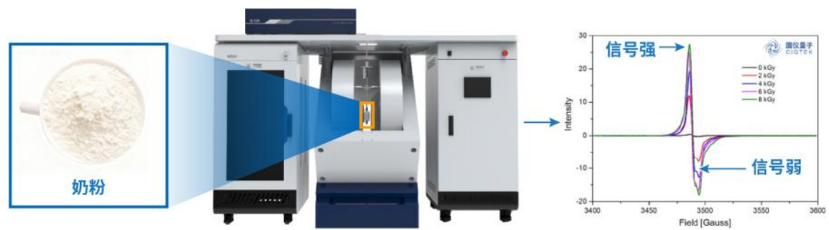
食品辐照可以延长食品保藏时间。以食品辐照为例，奶粉辐照杀菌后会产生自由基。 通过EPR可以精准评估食品辐照计量:确保达到预设的杀菌效果,在安全灭菌的同时,最大限度保留食品的营养。
