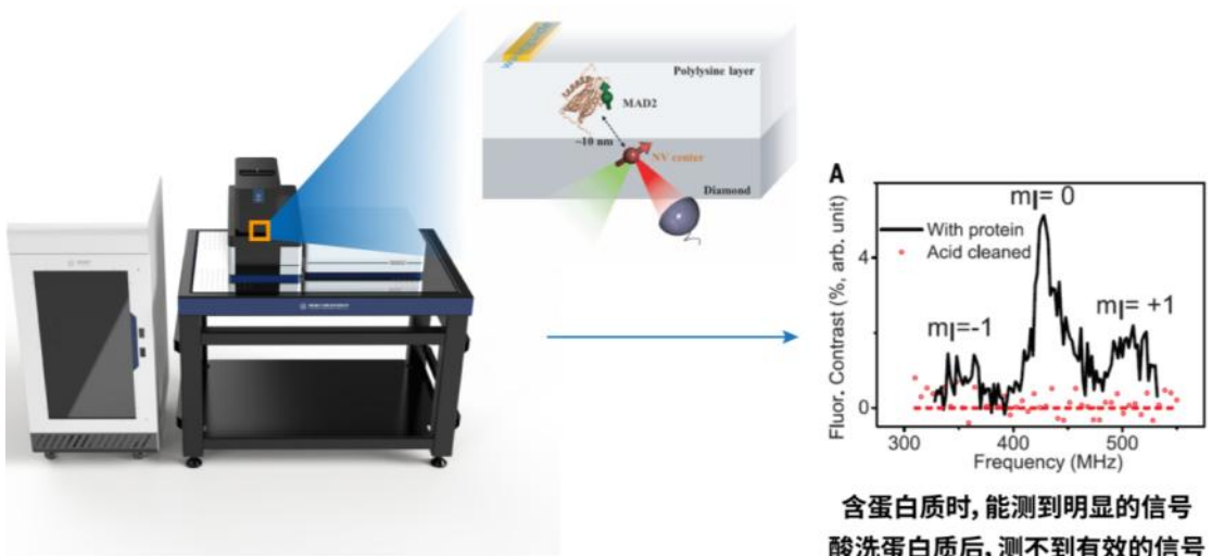
量子钻石单自旋谱仪应用示意图（以检测蛋白质分子为例）
