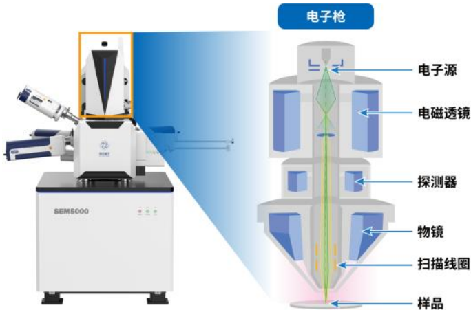
扫描电镜的结构示意图
