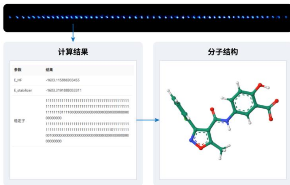
离子阱量子计算机应用示意图（以模拟分子结构为例）
