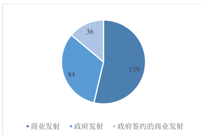
2024 年全球轨道发射次数构成（按发射类型）
