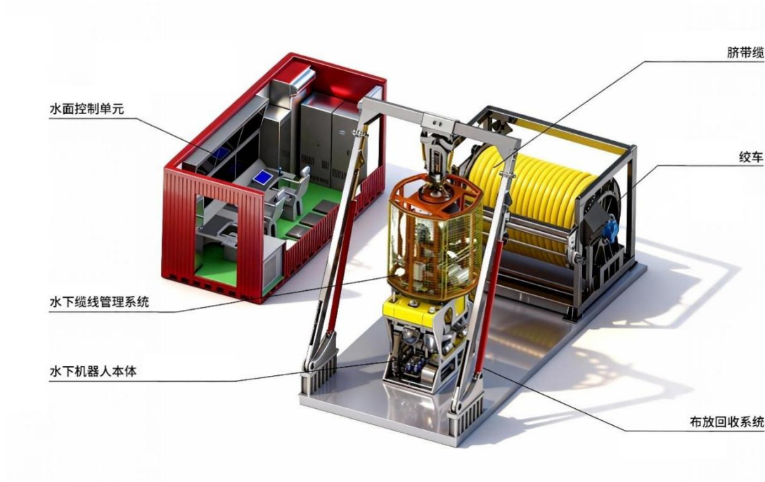
图：缆控水下机器人系统构成
