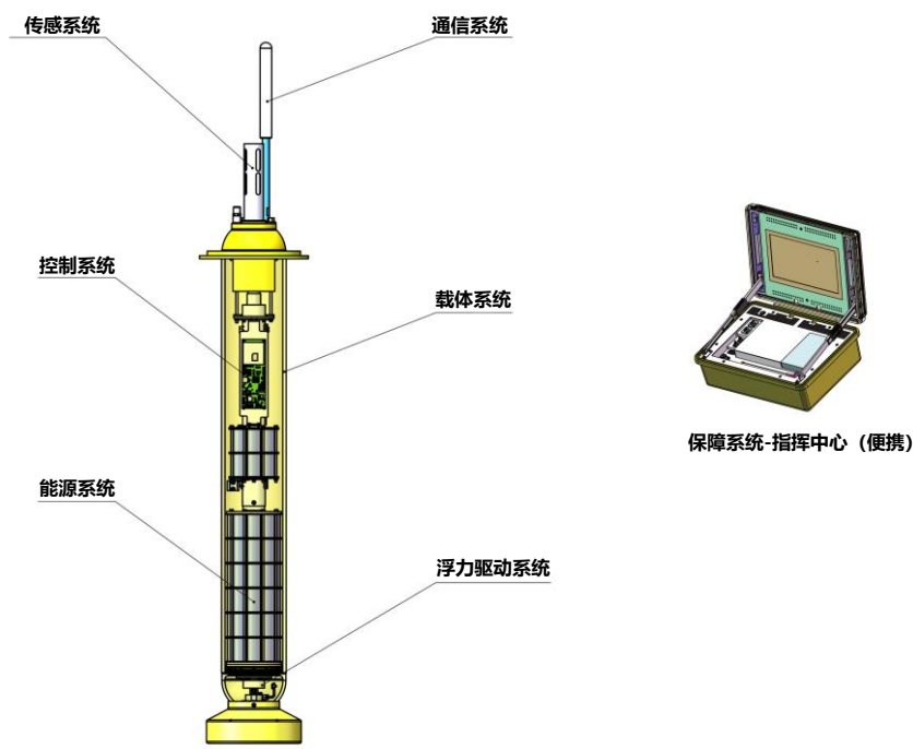
图：自动剖面浮标系统构成
