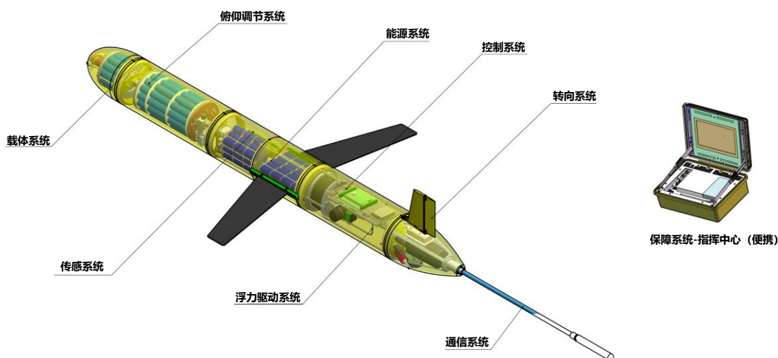
图：水下滑翔机系统构成
