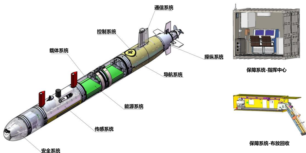
图：自主水下航行器系统构成
