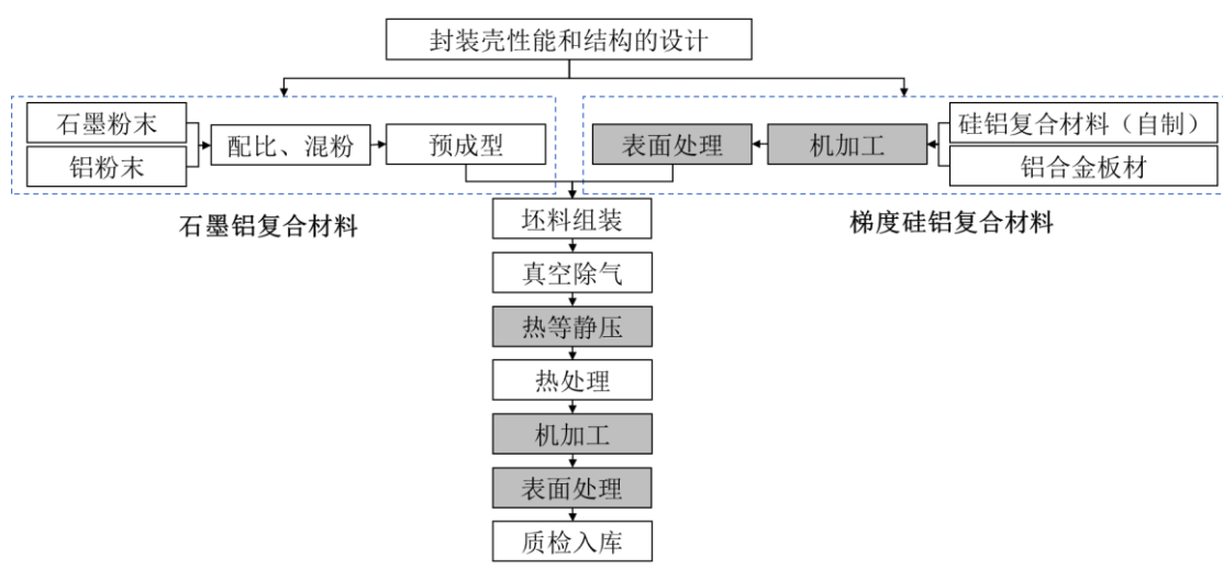
(2) 结构功能一体化复合材料生产工艺流程图
