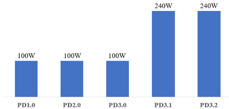
历代USB PD标准的功率传输范围
