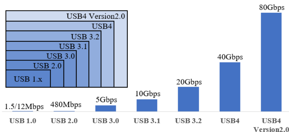
历代USB标准的通信速率和包含关系
