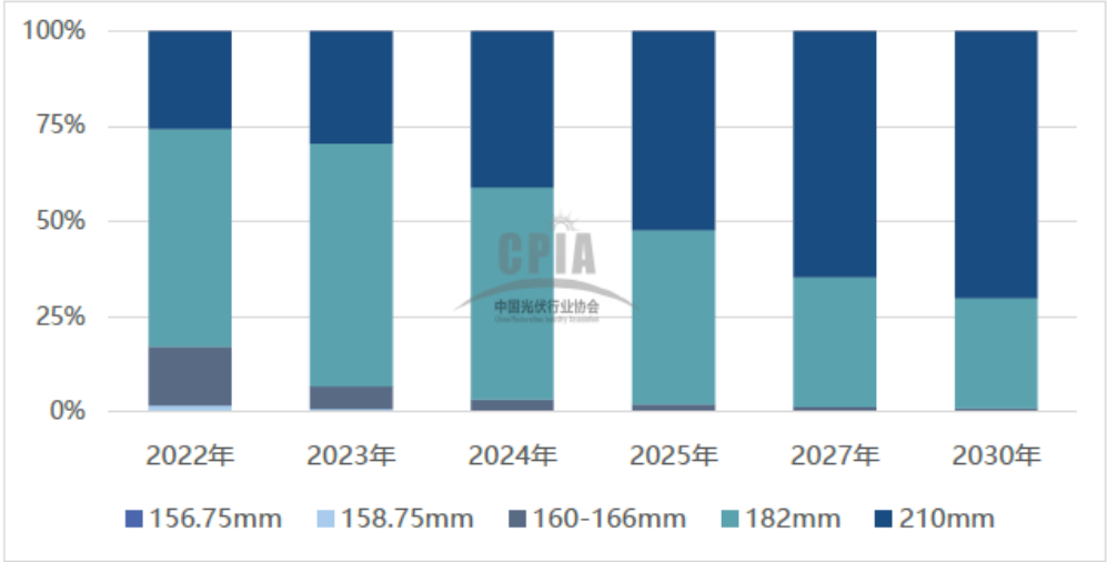
2022-2030 年不同尺寸硅片市场占比变化趋势统计图
