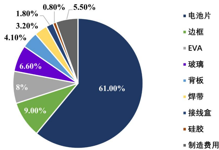
光伏组件成本结构统计图
