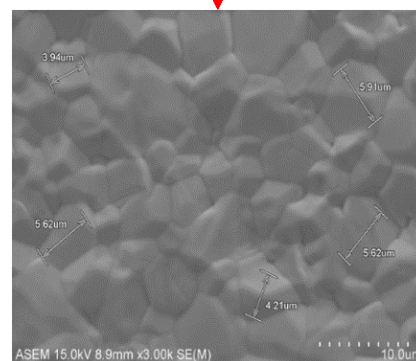
电子显微镜下引脚表面致密的镀层
