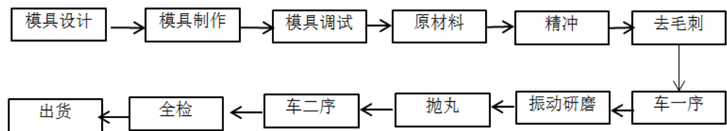
6）电驱动系统零部件生产工艺流程图
