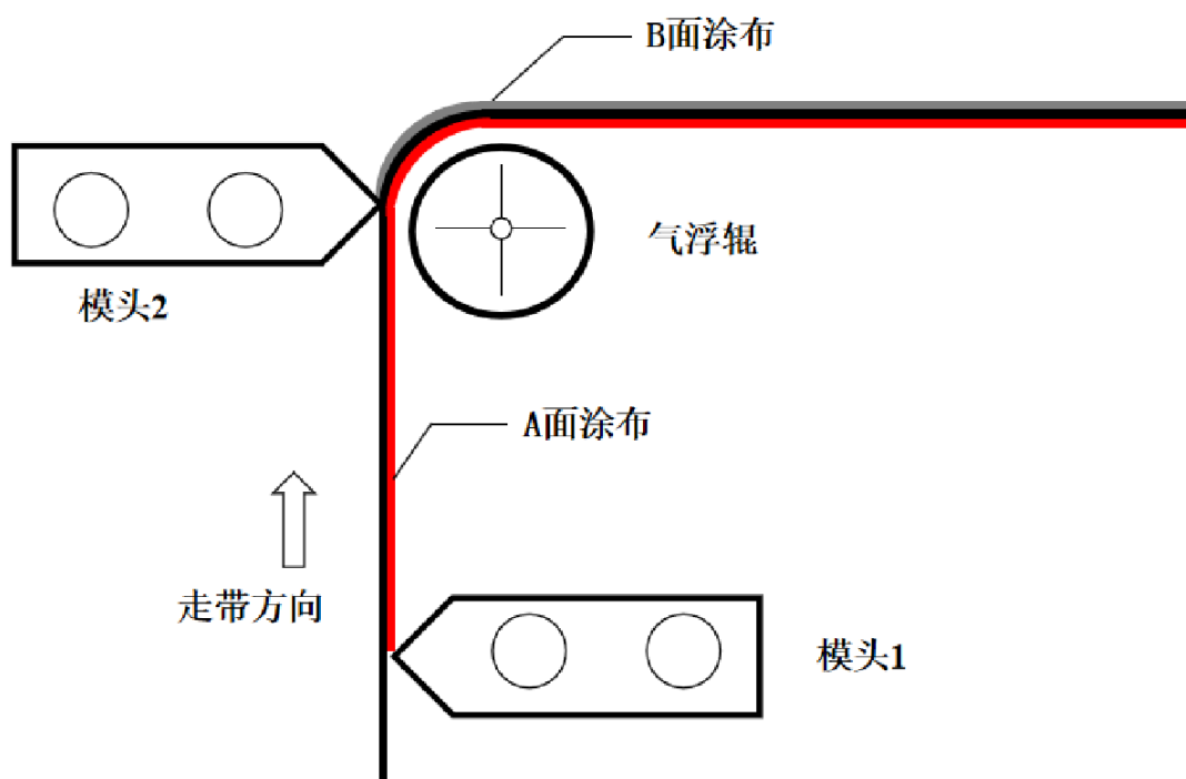
C.国内双面涂布技术原理图
