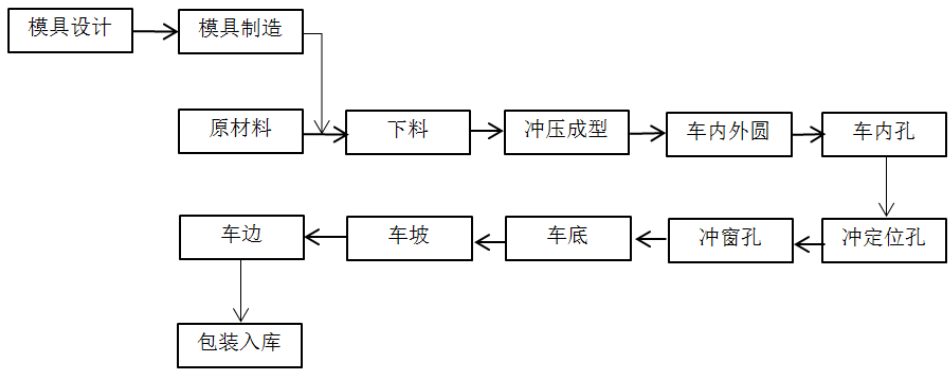
4）齿轮箱轴承保持架生产工艺流程图
