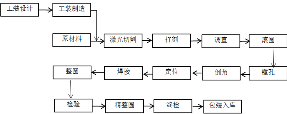
4）齿轮箱轴承保持架生产工艺流程图
