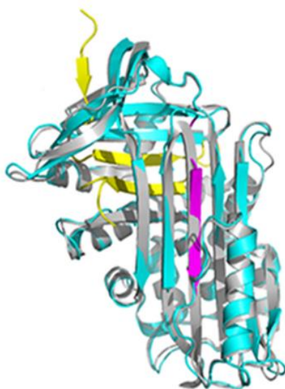
HY1003（蓝色）与人血 \alpha -1 抗胰蛋白酶（pAAT，灰色）晶体结构叠加图
