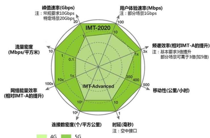
图：5G 与 4G 关键能力对比
