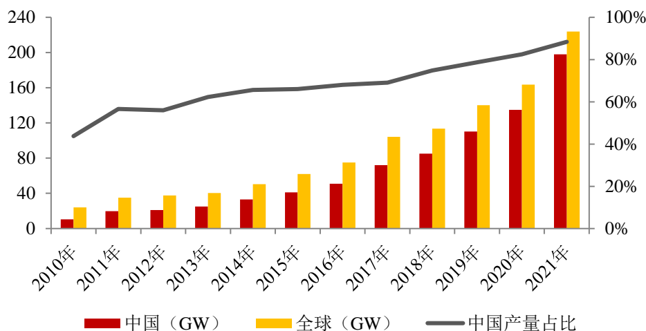
2010-2021年全球和中国电池片产量
