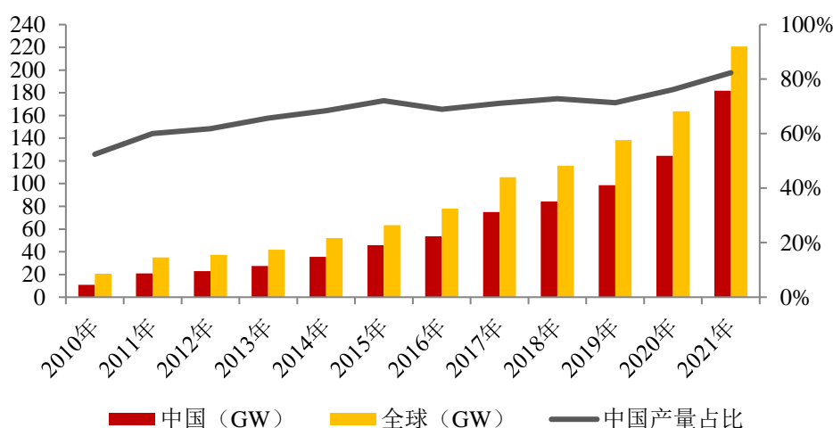
2010-2021年全球和中国组件产量
