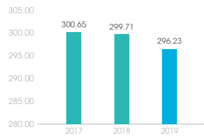
供电煤耗 (克标准煤/千瓦时)
