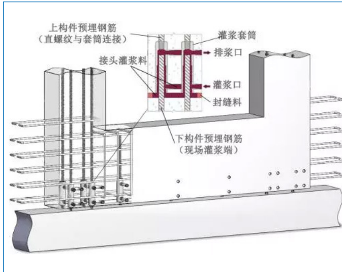
▶ 夹心保温立面节点详图
