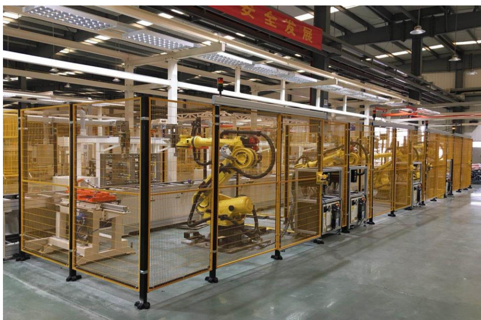
华域智能装备科技有限公司设计的副车架智能化装配线
