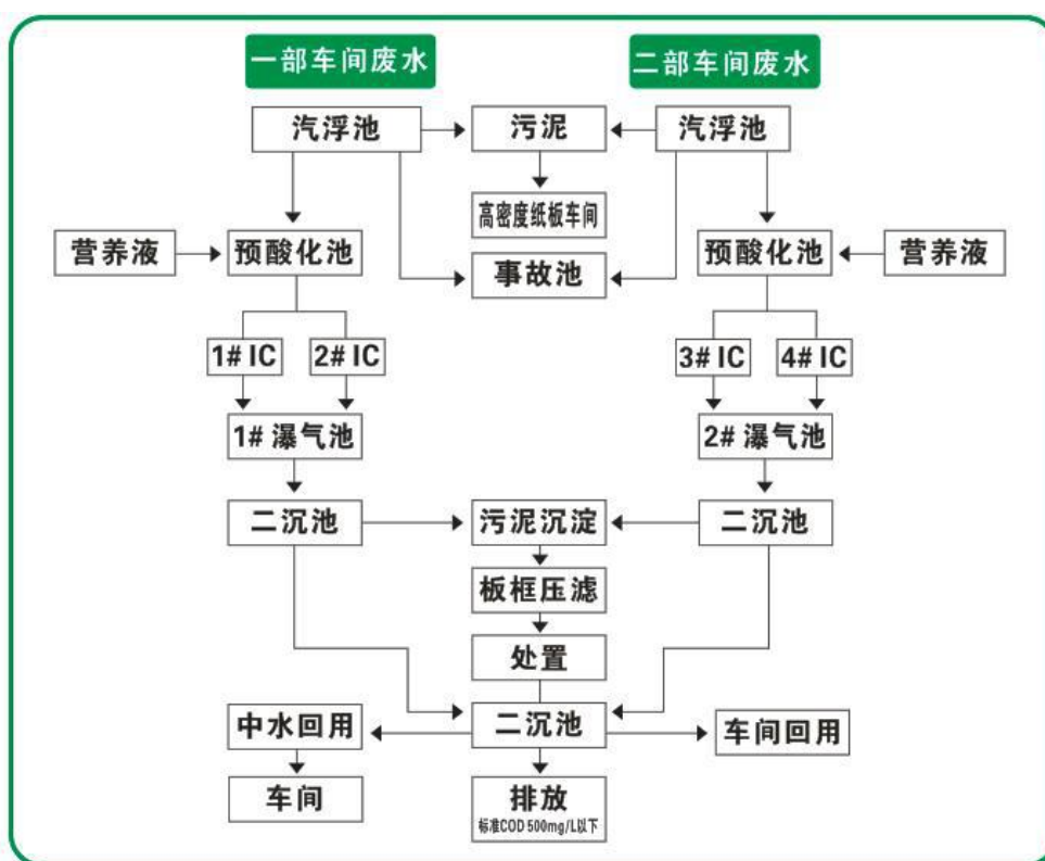
图 2：污水站流程图
