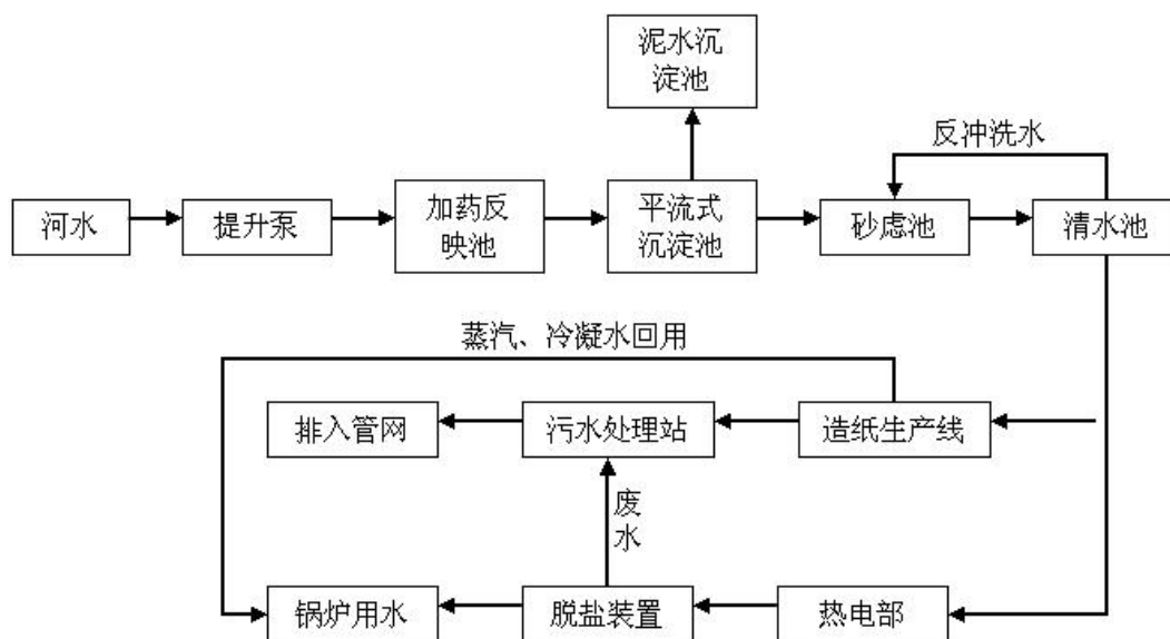
图 1：废水排放示意图
