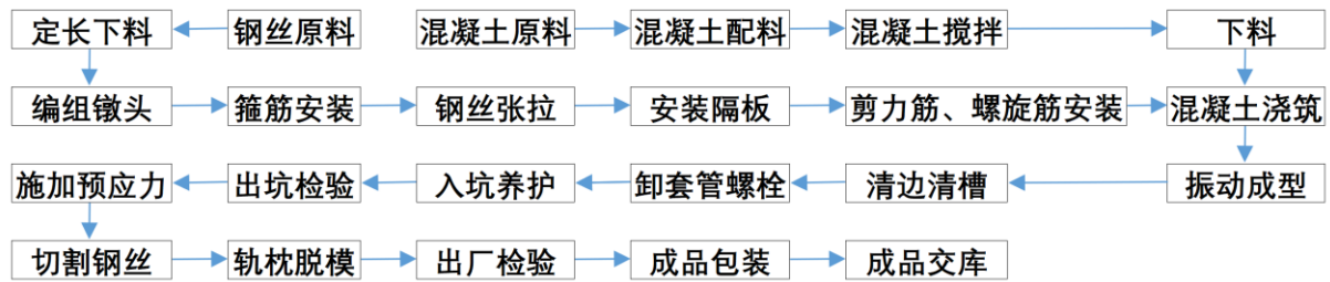
轨枕工艺流程图
