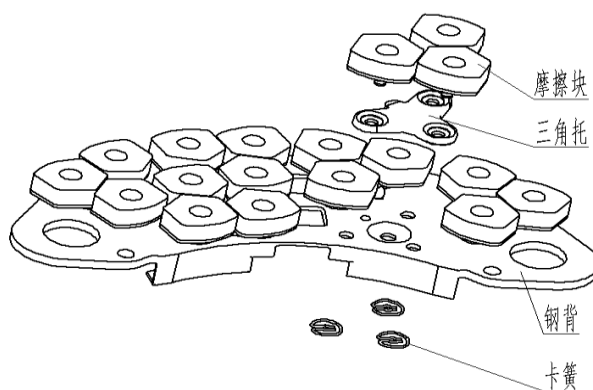
TS355 闸片结构与外形示意图
