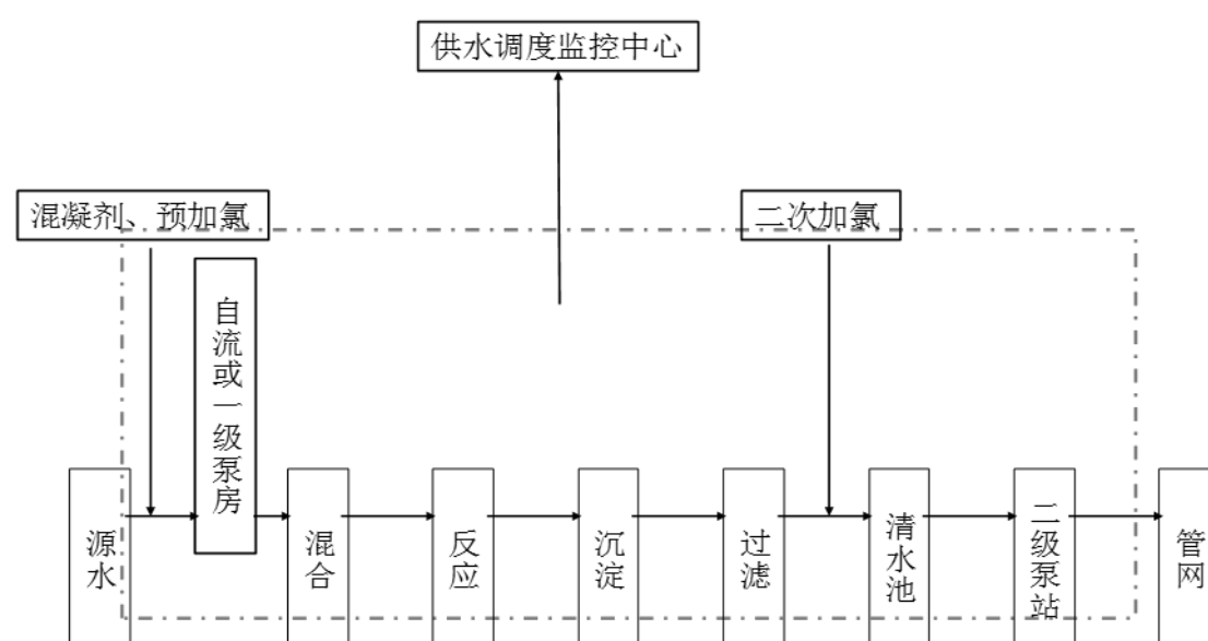
启迪桑德自来水生产工艺流程图
