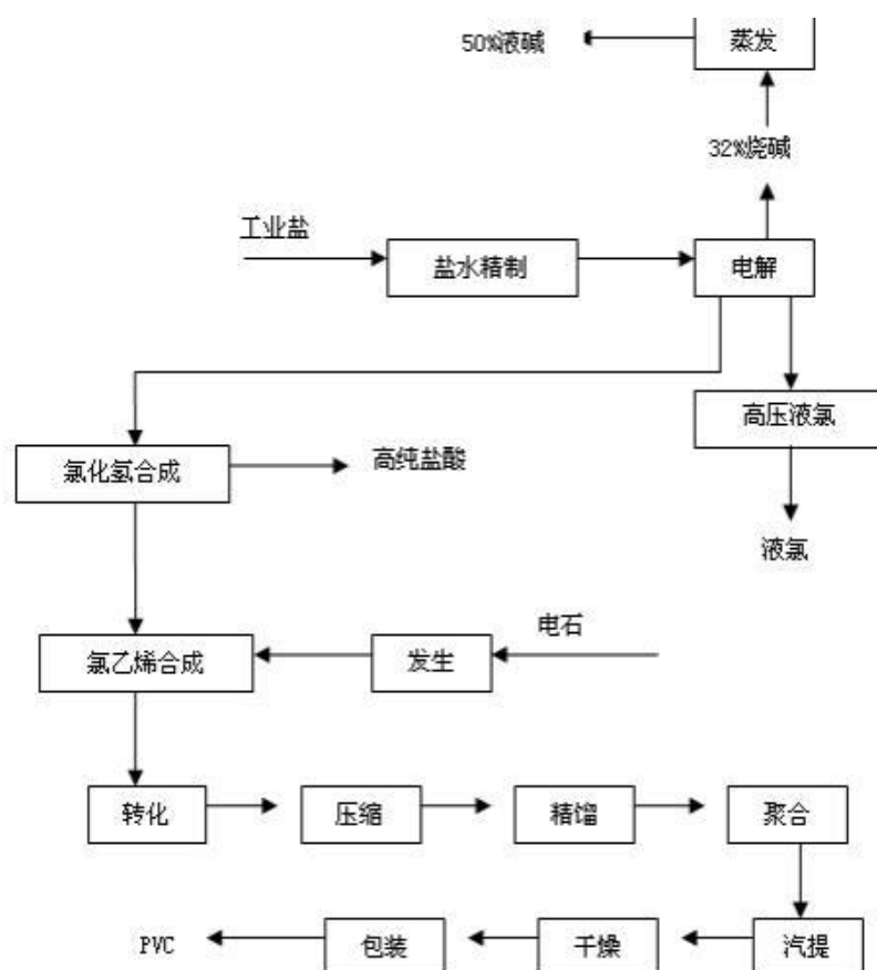
图：烧碱和 PVC 生产工艺流程图
