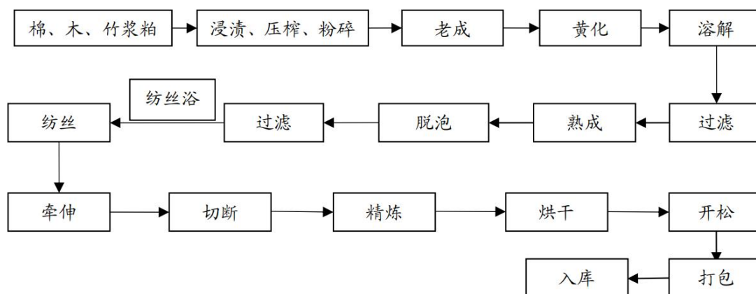
图：粘胶短纤维生产工艺流程图
