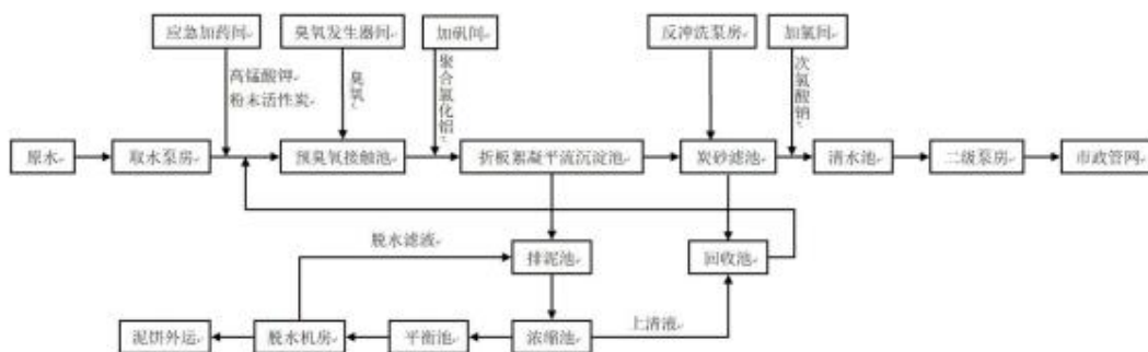
江南水务制水工艺流程图
