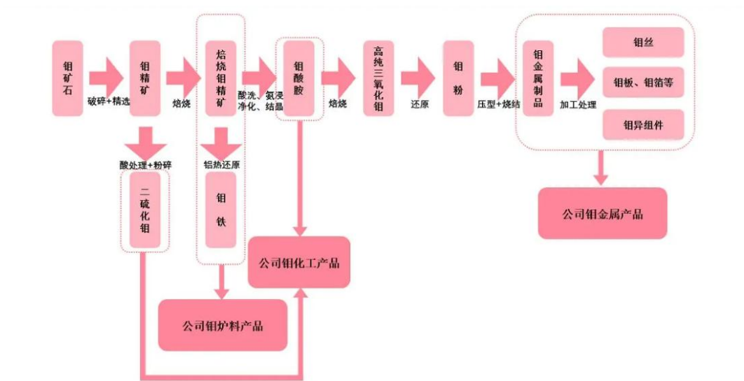
图:公司三大系列钼产品总生产步骤简析
