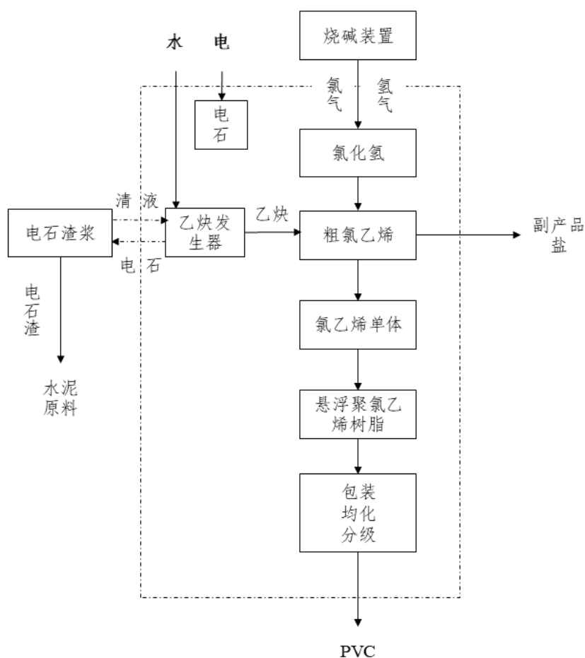
图：电石乙炔法
