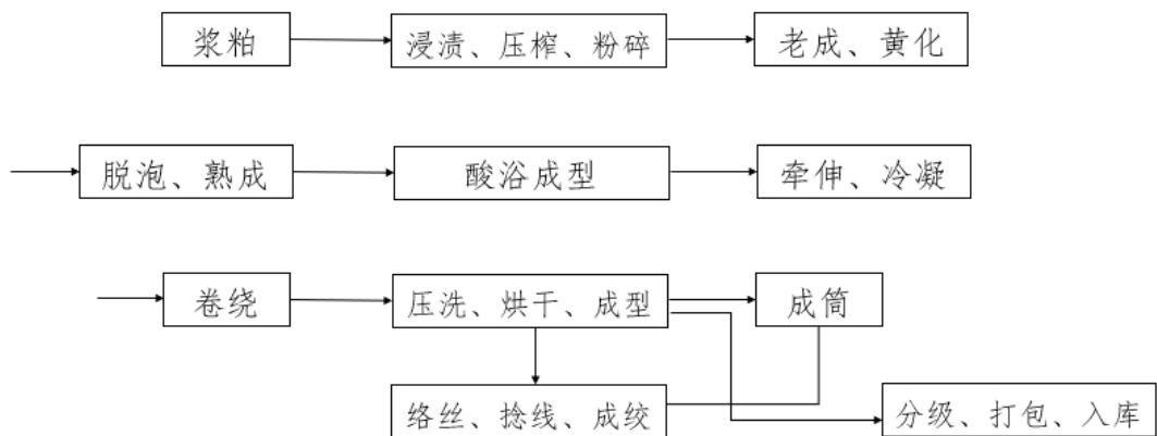
粘纤长丝生产工艺流程图
