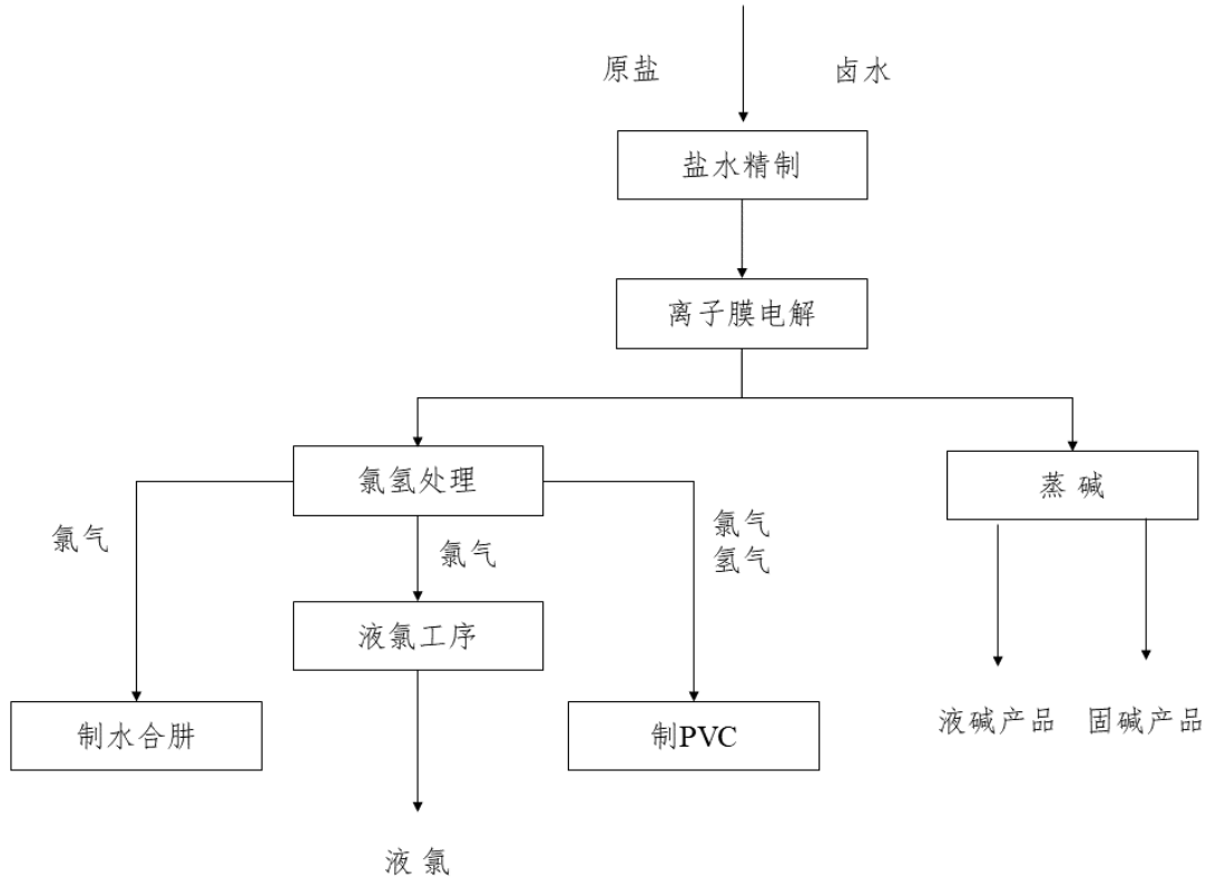
图：离子膜法制烧碱工艺
