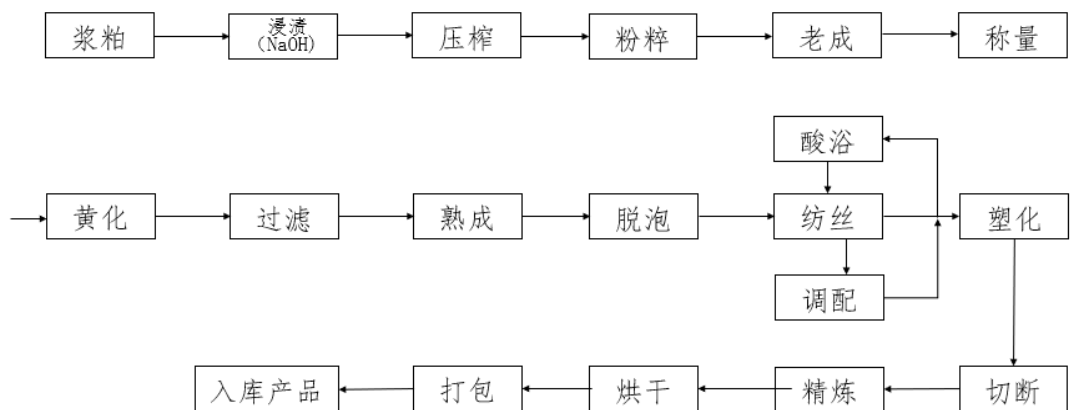
粘纤短丝生产工艺流程图
